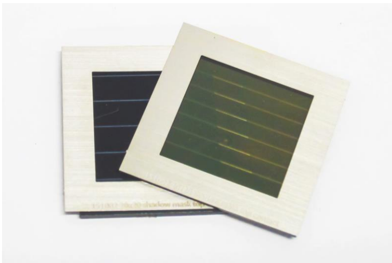
Prototypen der Tandem-Solarmodule, bestehend aus einem semitransparenten Perowskit-Solarmodul (rechts/vorne) und einem CIGS-Solarmodul (links/hinten). (Bild: imec/ZSW/KIT)
